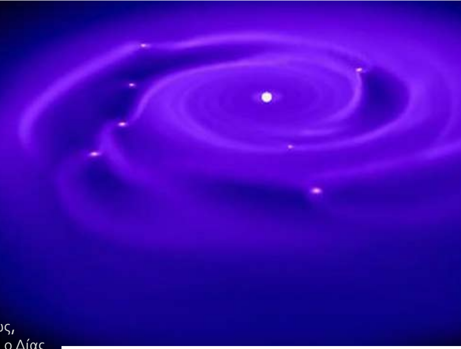
Προσομοίωση σχηματισμού αέριων γιγάντων, σύμφωνα με την θεωρία της αστάθειας δίσκου [φωτογρ. Mayer L., Quinn T., Wadsley J., Stadel J., "Formation of Giant Planets by Fragmentation of Protoplanetary Disks", Science 298, 1756-59 (2002)].
